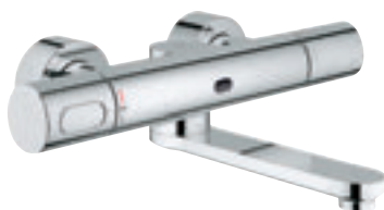
36 333 000 Infrarood elektronische thermostatische wastafelkraan sprong 251 mm
